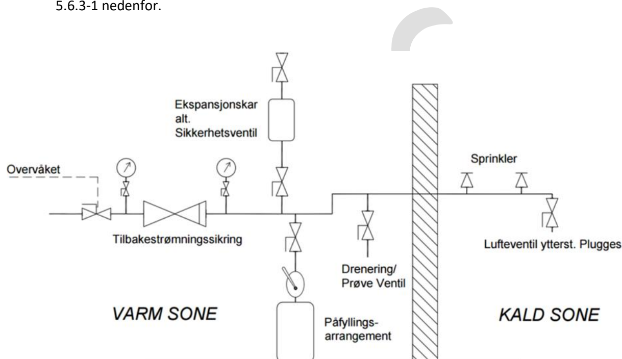
Figur 5.6.3-1: Oppbygning av kontrollventilsett for del av anlegg med frostvæskeblanding.
